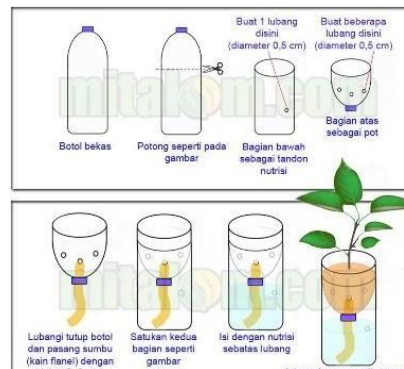
Metode Rakit Apung
