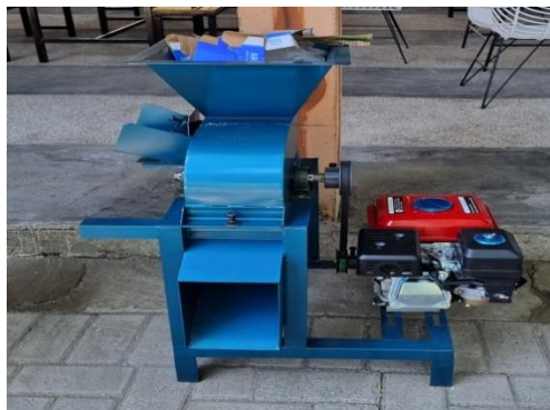
Gambar 7: TTG Mesin kompos
